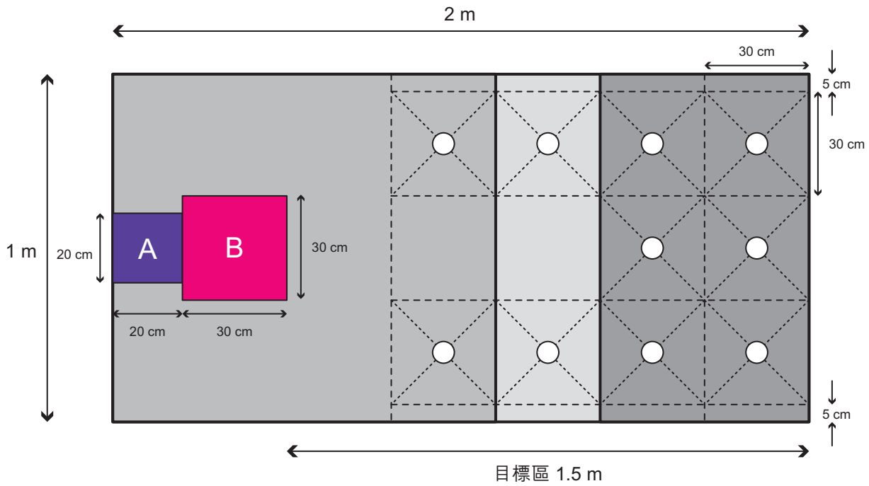
(俯視圖)
